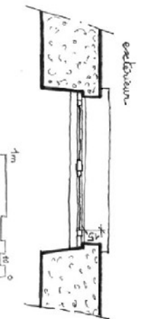
Pose en feuillure d'une menuiserie dans une baie.
