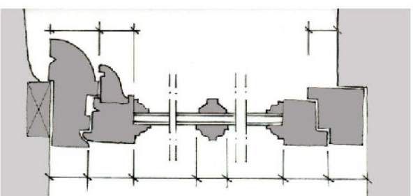
Coupe de détail (échelle 1/2 ou 1/1)
