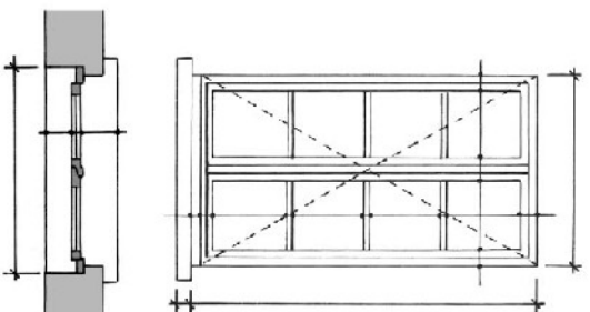
Élévation et plan (échelle 1/10e)
